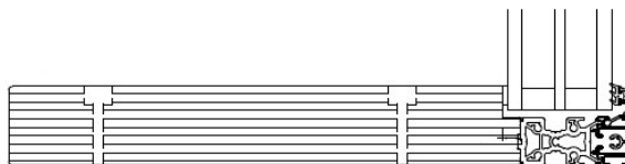
Snittegning - fast glas og kertokarm
